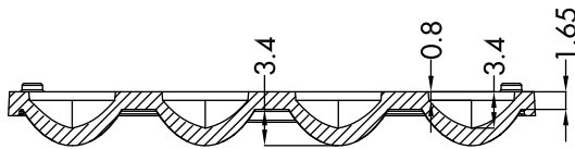
SECTION A-A
