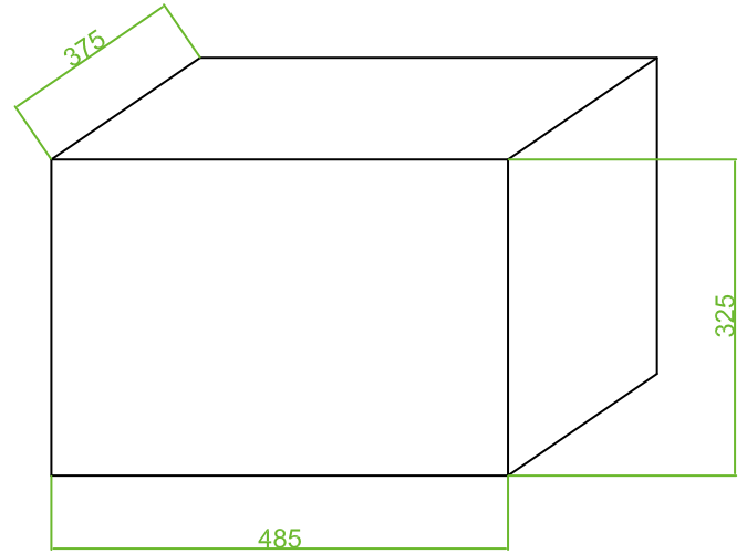
外盒 Cardboard Box-485*375*325
